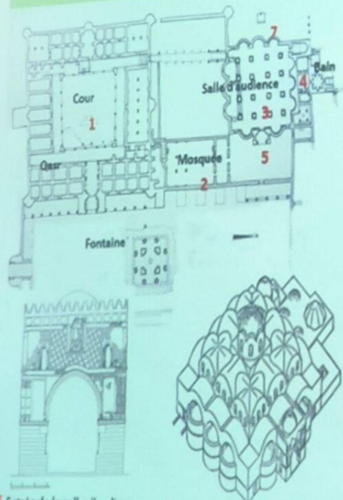
6 Recouvrement de la salle d'audience
